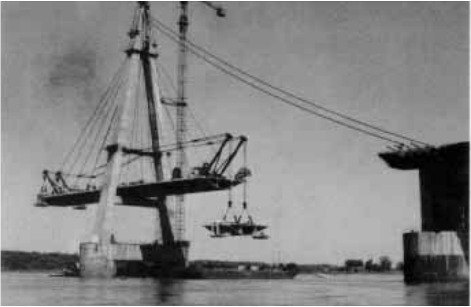
Fig. 43. Erection of Posadas Encarnacion Bridge, Argentina.
